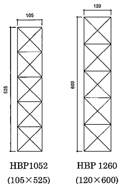
図 4.1 製品断面図
