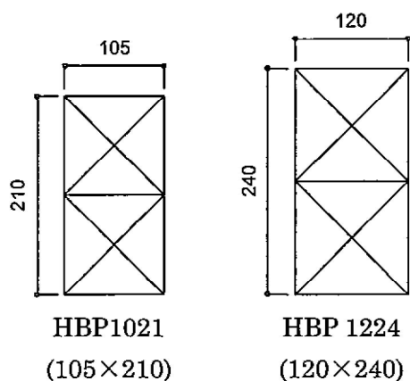
図 4.1 製品断面図
