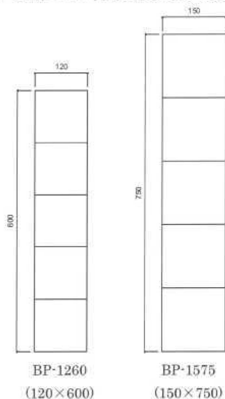
図 4.1 製品断面図
