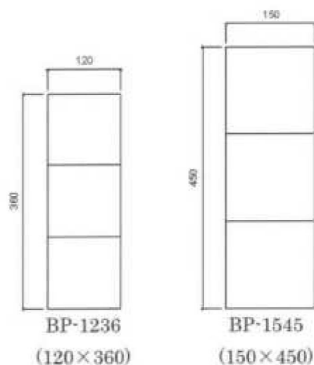
図 4.1 製品断面図
