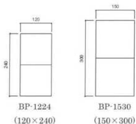
図 4.1 製品断面図
